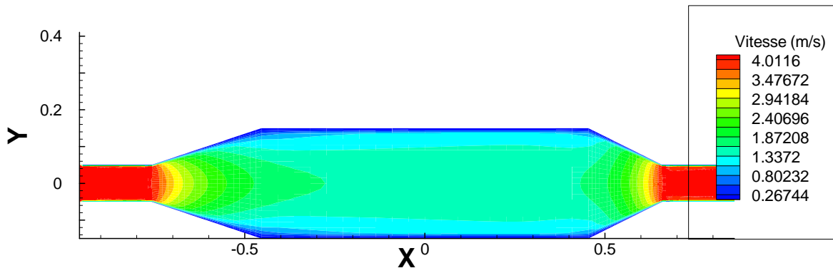
Figure 6 : Simulation numérique des vitesses à l'intérieur de la chambre d'empoussièremment
